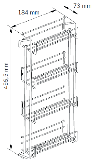
Полка для 12 банок, 184 мм.
