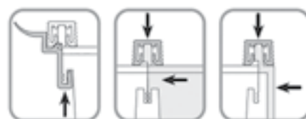
Схема установки соединительного профиля:
