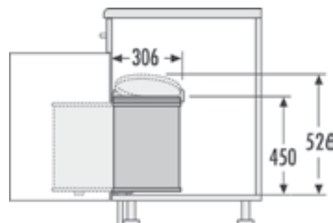
Схема и размеры корпуса:
