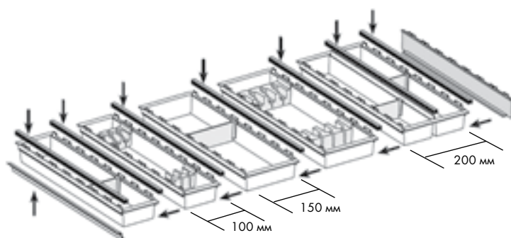
Схема сборки лотка:
