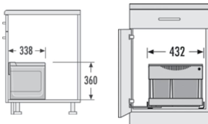
Схема и размеры системы:
