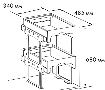
Размеры вёдер:
