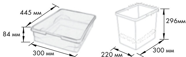
Размеры ведра и лотка:
