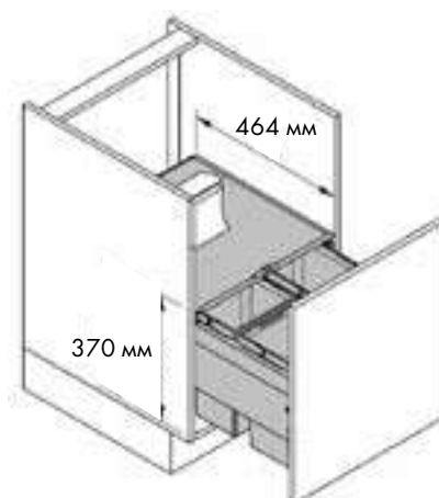
Схема и размеры корпуса:
