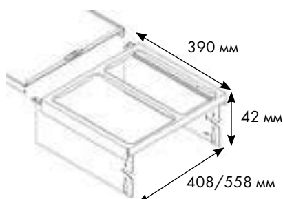
Размеры рамы:
