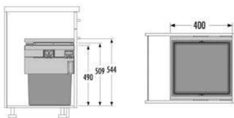
Схема и размеры системы:
