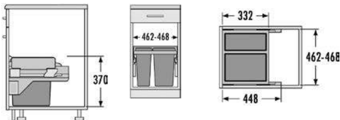
Схема и размеры системы:
