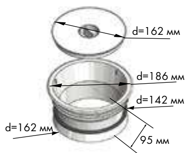
Схема и размеры модели под пакет:
