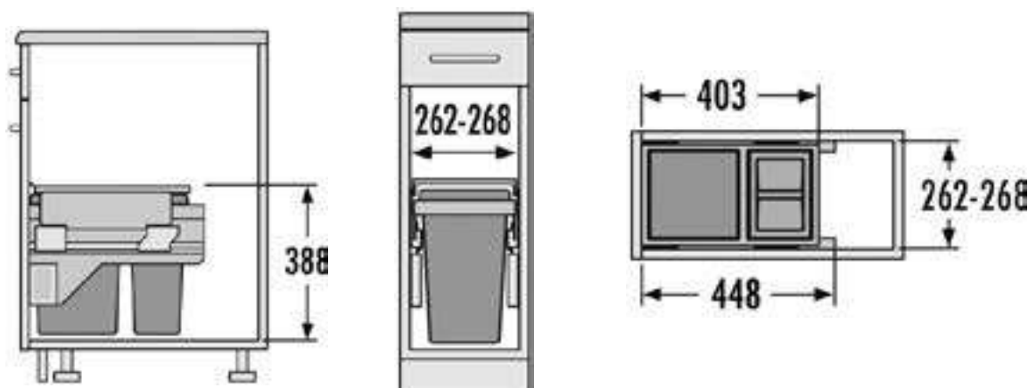
Схема и размеры системы:
