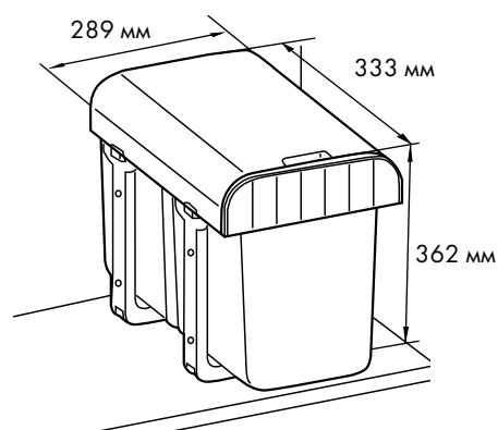
Размеры ведра:
