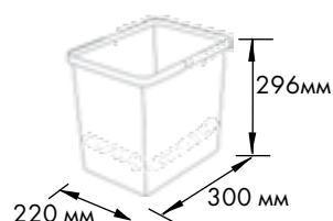
Размеры вёдер:
