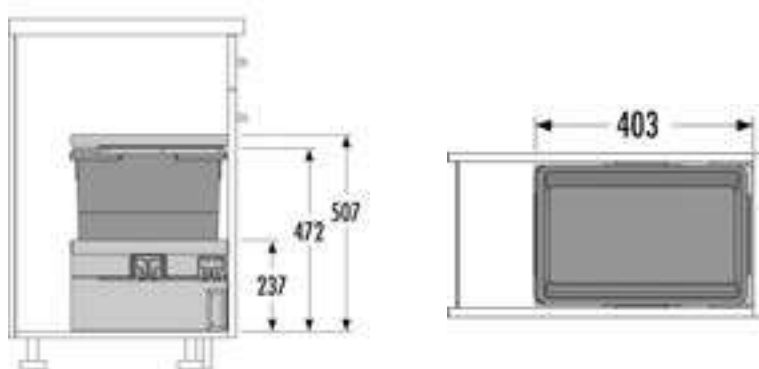
Схема и размеры системы:
