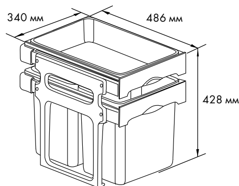
Размеры ведра и лотка:
