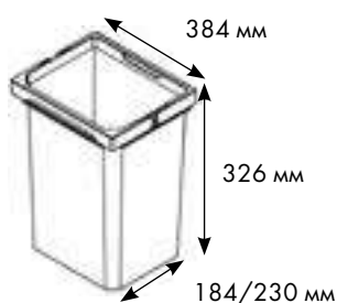
Размеры ведра:
