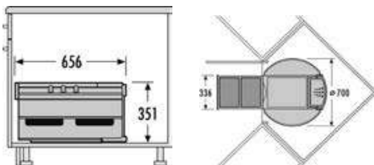
Схема и размеры системы:
