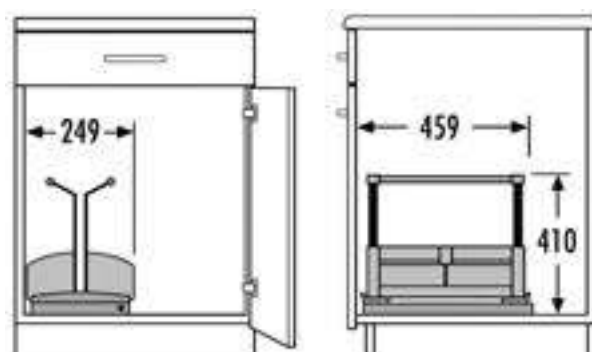
Схема и размеры системы:
