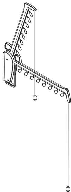
ОТТО лифт для навески одежды Otto, настенный
