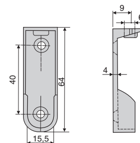
держатель штанги 15x30, с боковым и верхним креплением
