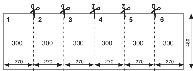
Примеры раскроя коврика для ящиков.
