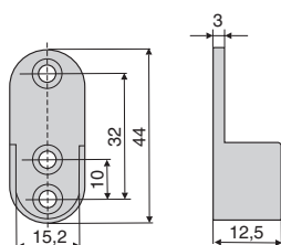
держатель штанги 15x30, с боковым креплением
