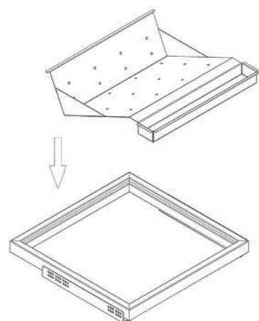
BM.041 поддон для обуви H=131
