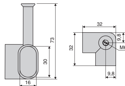
держатель штанги 15x30, угловой с верхним креплением
