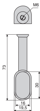
держатель штанги 15x30, торцевой с верхним креплением
