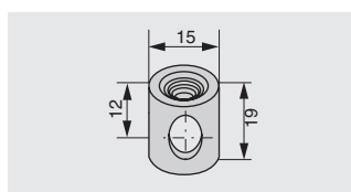
бочонок для стяжки конической XS, d.15 мм, h.19 мм, M10
