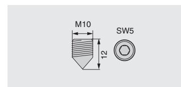
винт для стяжки конической XS, M10x12 под ключ Ch.5
