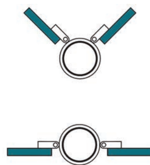
Вариант внутреннего крепления
