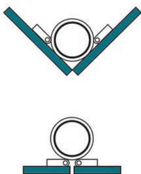
Вариант внешнего крепления
