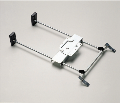
механизм для вставки стола (поворотный)
